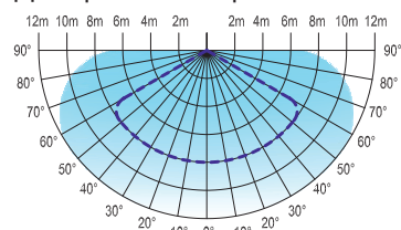
Диаграмма направленности датчиков движения
