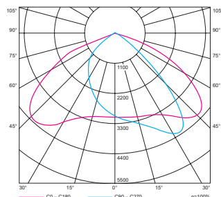
ДКУ 1002Ш, ДКУ 1004Ш
