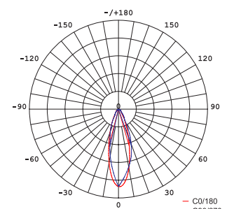
КСС К (30°)
