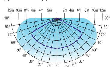
Диаграмма направленности датчиков движения
