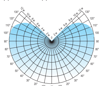
Диаграмма направленности датчиков движения
