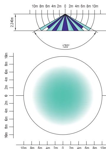
Диаграмма направленности датчиков движения
